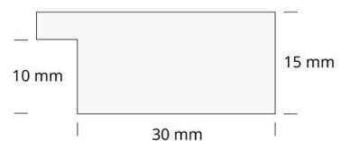
Sezione cornice dimensioni reali Frame section real sizes
